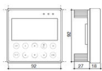
DIRIS Digiware D-40/D-50/D-70
