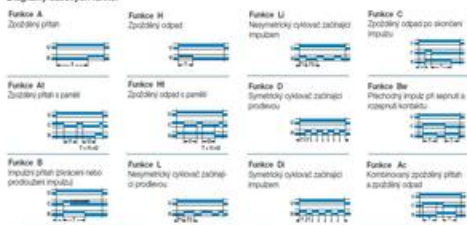
Diagramy časových funkcií
