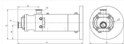
Mäz HYGHSPIN Extended kompaktnonrad (mm)
