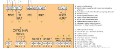
Svorky a zapojení
